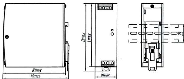
Fig.1: Dimensiones del producto, los valores están detallados en la Tabla 2 .
