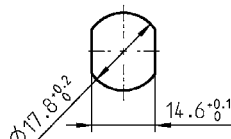
Corte para fijación con clip
