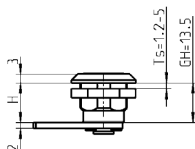
Corte para fijación con tuerca
