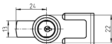
Fijación con clip
