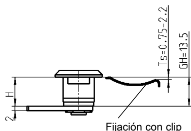
Corte para fijación con clip
