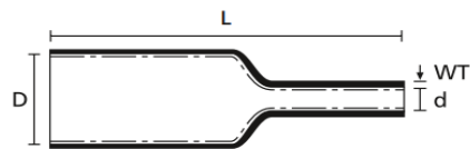
Tubo Termorretráctil 4:1 con Adhesivo
