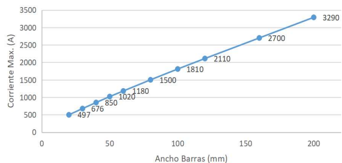
Capacidad de corriente en barras de cobre de 10mm de grosor con \Delta T=40^{\circ}C , segun DIN 43671
