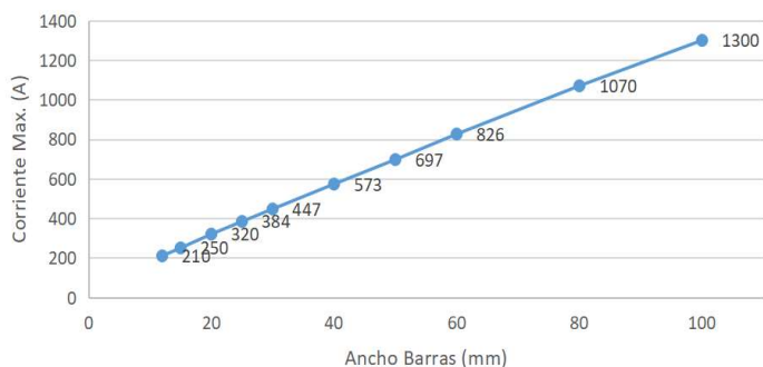
Capacidad de corriente en barras de cobre de 5mm de grosor con \Delta T=40^{\circ}C , segun DIN 43671
