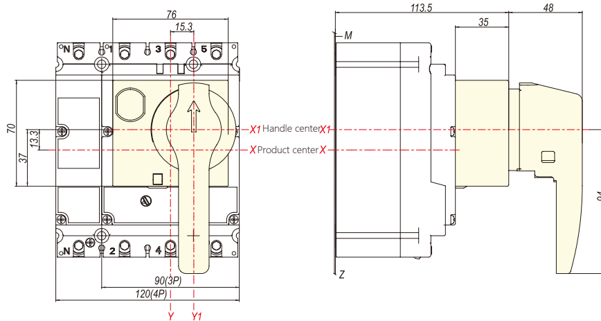
Dimensiones DRH21-M8 / 072204021CH
