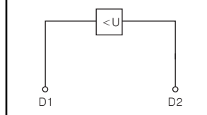
Esquema de conexión Bobina de mínima tensión
