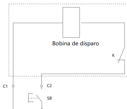
Esquema de conexiones
