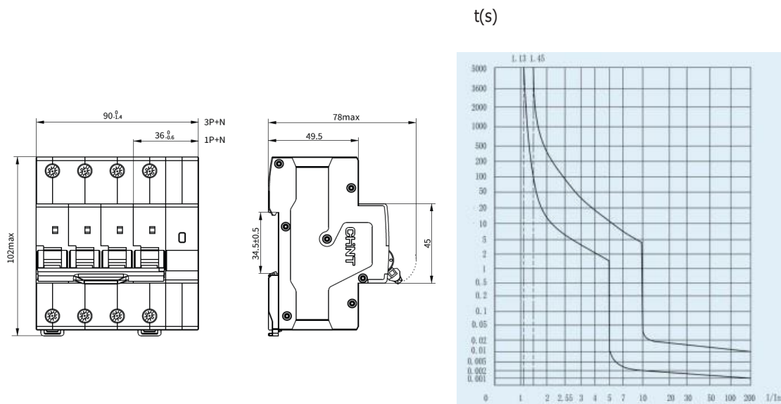
Curva C
