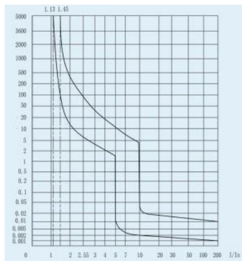
Curva C
