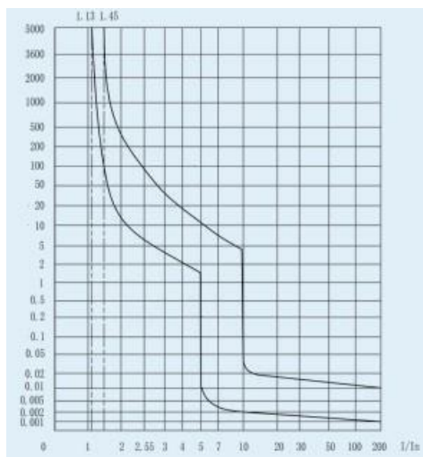
Curva C
